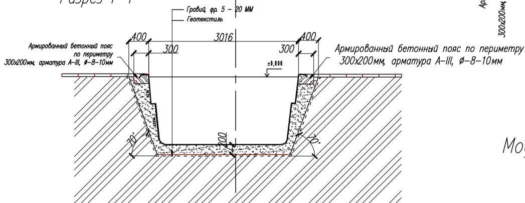
Разрез 1-1
